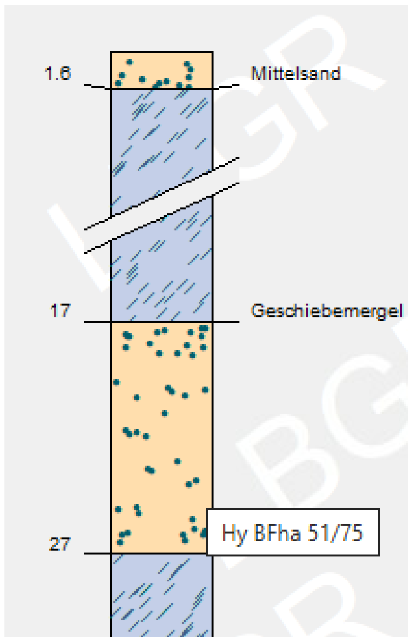
Abb. 1: Vorprofil GWM Börnicke 1/26
